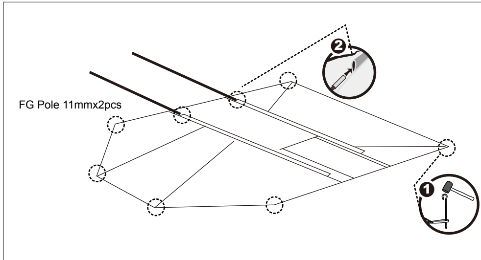
Flysheet
